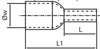
Рисунок 1. Наконечники-гильзы втулочные типа Е
